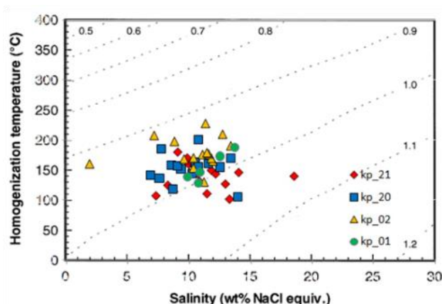
شکل ۱۷ نمودار دمای همگن شدن نسبت به شوری برای میانبارهای سیال نمونه های مورد بررسی. خطوط چگالی بر پایه رابطه مرجع [۲۷] و نرم افزار FLINCOR محاسبه شده اند. چگالی میانبارهای سیال حدود ۱ گرم بر سانتی متر مکعب است که نشان می دهد که فاز سیال در زمان به دام افتادن به صورت مایع بوده است.
