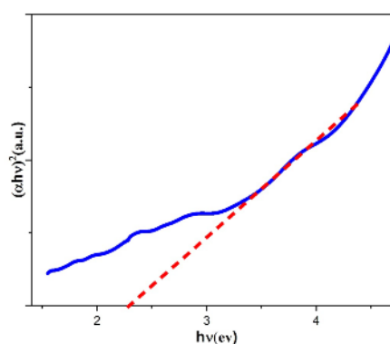
شکل ۵ نمودار (\alpha h\nu)^2 نسبت به h\nu برای فریت بیسموت بدون روکشگر.
