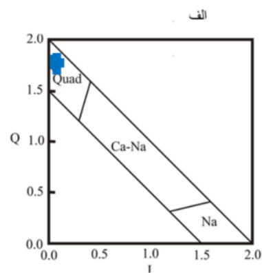
شکل ۷ الف) نمایش ترکیب شیمیایی پیروکسن‌ها در نمودار (Q-J ب) جایگاه پیروکسن‌ها در نمودار مثلثی Wo-En-Fs [۱۴].
