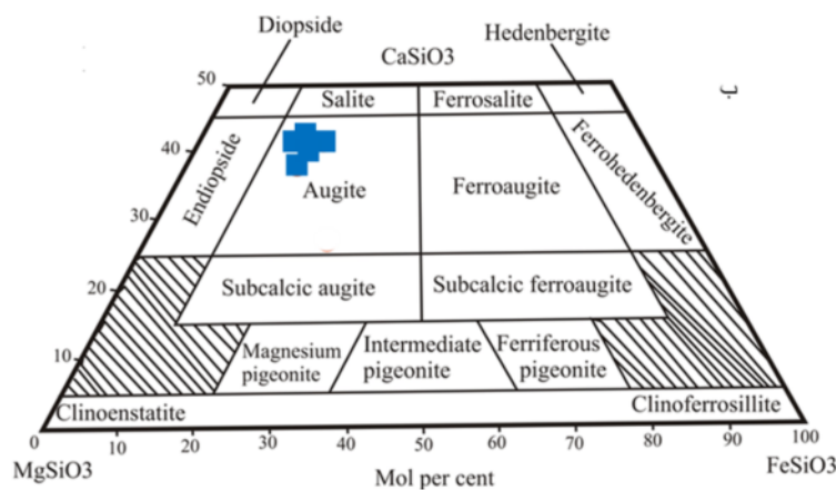
شکل ۷ الف) نمایش ترکیب شیمیایی پیروکسن‌ها در نمودار (Q-J ب) جایگاه پیروکسن‌ها در نمودار مثلثی Wo-En-Fs [۱۴].
