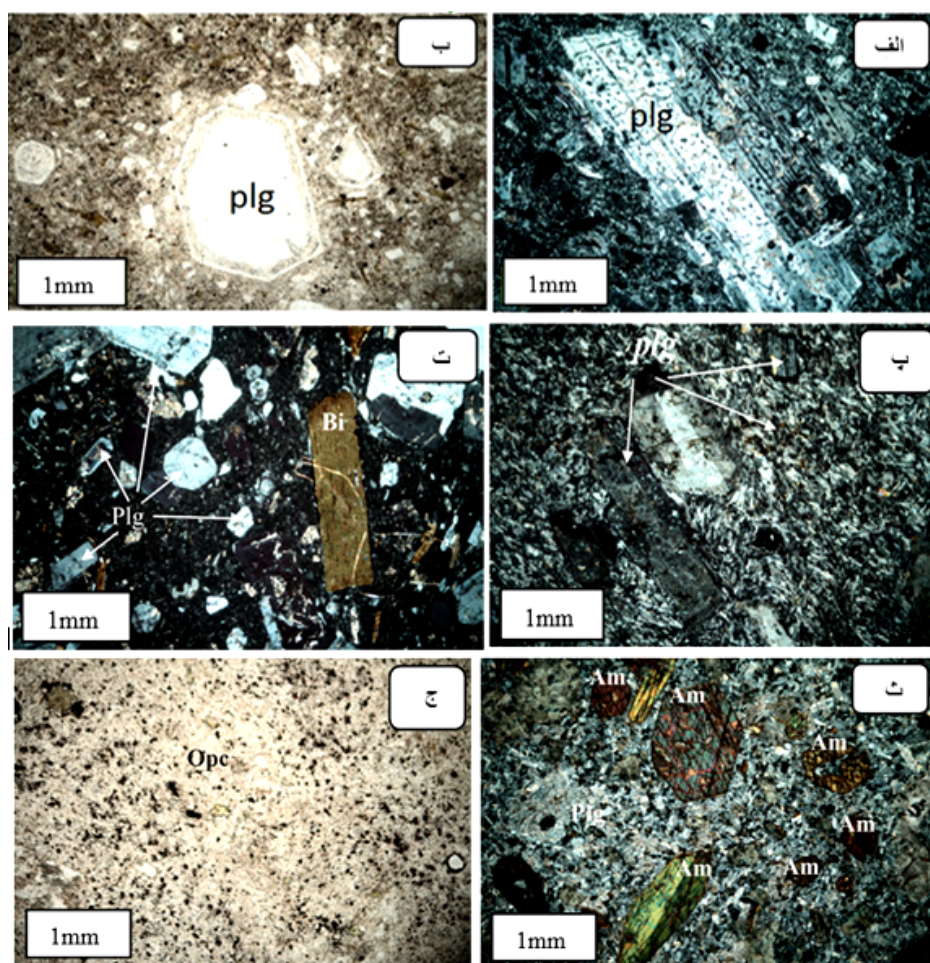
شکل ۳ تصویرهای میکروسکوپی در نور قطبیده متقاطع، XPL (الف-ث) و نور قطبیده صفحه‌ای، ppl (ج). (الف-ب) بافت انحلالی (غریالی) در درشت بلورهای پلاژیوکلاز (ب) شکل گیری پوشش‌های غبارآلود پیرامون پلاژیوکلاز، (پ) بافت جریان‌ی (ت) کانی بیوتیت و پلاژیوکلاز (ث) کانی آمفیبول بدون ماکل و با ماکل دوتایی به همراه بلورهای ریز کانی پلاژیوکلاز (ج) پراکندگی کانی‌های کدر در سنگ‌های داسیتی منطقه (Plg): پلاژیوکلاز؛ Bi: بیوتیت؛ Am: آمفیبول و Opc: کانی کدر).
