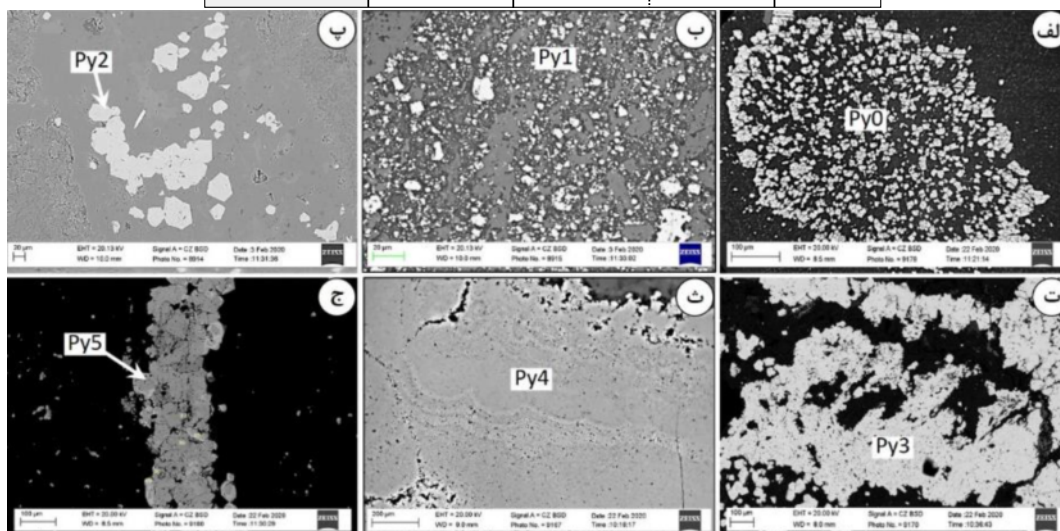
شکل ۵ توالی هم‌مرزایی مجموعه کانی‌ها و جایگاه انواع مختلف پیریت الف تا ج) همراه با تصاویر میکروسکوپ الکترونی در کانسار طلای زرشوران.
