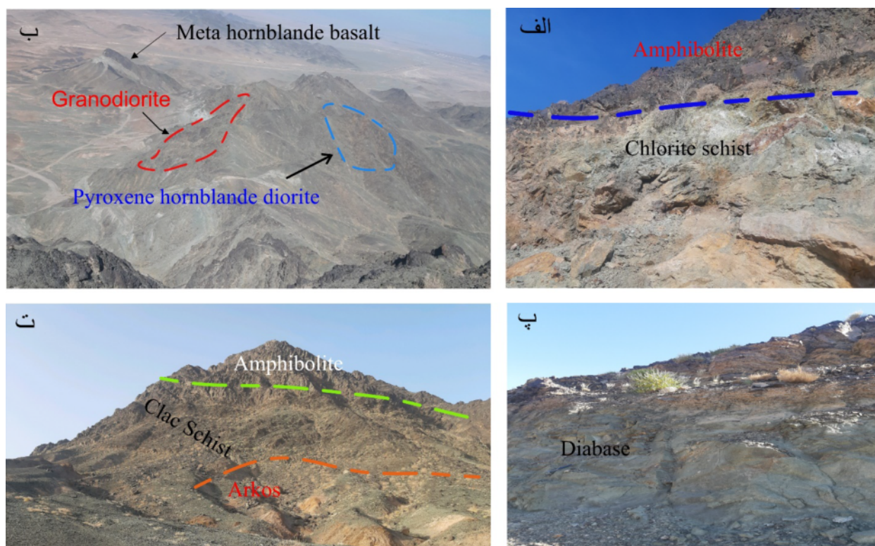
شکل ۲ تصاویر صحرایی از واحدهای سنگی منطقه اکتشافی سیاجک: الف) رخنمون‌های واحد سنگی آمفیبولیت (رنگ سفید)، کلریت شیست (رنگ سیاه) دید به سمت شمال، ب) متا هورنبلند بازالت (رنگ سیاه)، گرانودیوریت (رنگ قرمز)، پیروکسن هورنبلند دیوریت (رنگ آبی) دید به سمت شرق، پ) دیاباز (رنگ سیاه) دید به سمت غرب، ت) رخنمون واحد کالک‌شیست آهکی (رنگ سیاه)، آرکوز (رنگ قرمز)، دید به سمت شمال
