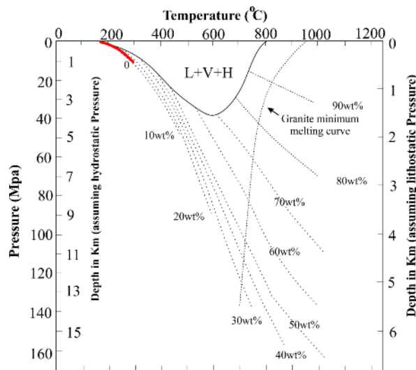
شکل ۱۰ نمودار فشار- دمای نشان‌دهنده رابطه فازها در سامانه H_2O-NaCl در فشارهای هیدروایستایی و سنگ ایستایی [۲۵]. L = مایع، V = بخار، H = هالیت. خط‌چین‌ها پربندهای ثابت درصد وزنی NaCl محلول در شورابه هستند. خط باریک خاکستری منحنی کمترین ذوب گرانیات را مشخص می‌کند. خط ضخیم مشکی مرز سه فازی، L+V+H را برای سامانه NaCl-KCl-H_2O با Na/K در محلول ثابت شده بوسیله آل بیت و فلدسپار قلیایی در دماهای مشخص نشان می‌دهد.
