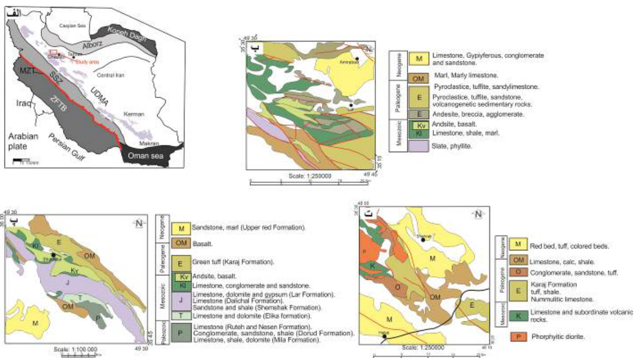
شکل ۱ الف) نقشه ساده شده زمین‌شناسی-ساختاری ایران [۱۳]؛ ب) نقشه ساده شده زمین‌شناسی منطقه نوبران [۱۴]؛ پ) نقشه ساده شده زمین‌شناسی منطقه آوج [۱۵]؛ ت) نقشه ساده شده زمین‌شناسی منطقه حلب [۱۳].
