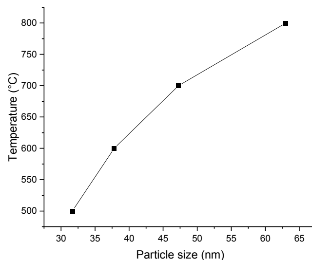
شکل ۲ تغییرات میانگین اندازه ذرات با دمای تکلیس.
