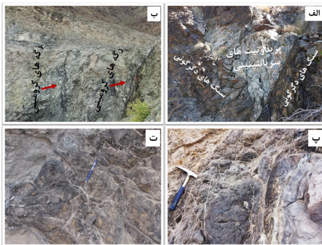
شکل ۴ (الف) واحد پریدوتیت سرپانتینیته شده به صورت گسله در کنار واحدهای دگرگونی، دید به سمت شمال شرق؛ (ب) رگه‌های سیاه کرومیت در سنگ‌های سفید دونیتی، دید به سمت شمال؛ (پ و ت) رگه‌های سرپانتینیته در واحدهای پریدوتیت، دید به سمت شمال غرب.
