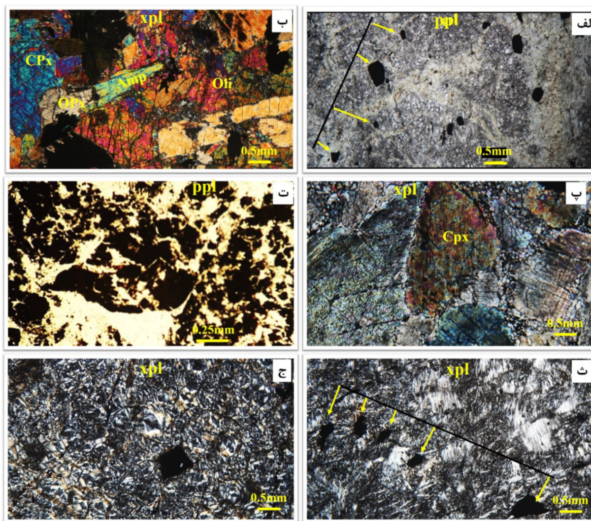
شکل ۶ تصاویر میکروسکوپی دونیت، ورلیت، پیروکسنیت، کرومیتیت و سرپانتینیت: الف) بلورهای شکل‌دار تا نیمه‌شکل‌دار کرومیت به صورت پراکنده و جهت‌دار در دونیت در نور قطبیده صفحه‌ای (PPL)؛ ب) شکفته‌بلورهای الیوین (Oli)، کلینوپیروکسن (CPX)، ارتوپیروکسن (OPX) و شکفته بلورهای آمفیبول (Am) در ورلیت در نور قطبیده متقاطع (XPL)، با بزرگنمایی 40x؛ پ) کانی‌های کلینوپیروکسن در پیروکسنیت در XPL با بزرگنمایی 40x؛ ت) کرومیتیت کروم اسپینل‌های بی‌شکل با آثار خردشدگی شدید، با رنگ نارنجی و قهوه‌ای تیره و دارای میانبره‌های سرپانتین که با رنگ سفید در PPL با بزرگنمایی 100x مشخص هستند؛ ث) کروم اسپینل‌های به‌صاف شده و ج) کروم اسپینل شکل‌دار در سرپانتینیت در XPL، با بزرگنمایی 40x.
