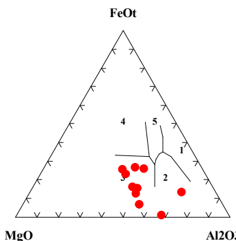
شکل ۱۰ نمودار \text{Al}_2\text{O}_3 , \text{MgO} , \text{FeOt} نمونه‌های مافیک و اولترامافیکی صحنه.
