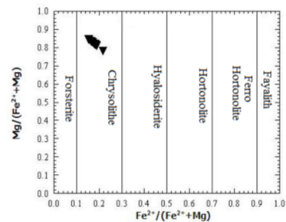
شکل ۳ ترکیب الیوین سنگ‌های گابرویی بر پایه نمودار \text{Fe}^{2+}/(\text{Fe}^{2+}+\text{Mg}) نسبت به \text{Mg}/(\text{Fe}^{2+}+\text{Mg}) .
