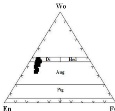
شکل ۵ ترکیب پیروکسن سنگ‌های گابرویی هرسین در نمودار مثلثی En-Fs-Wo.
