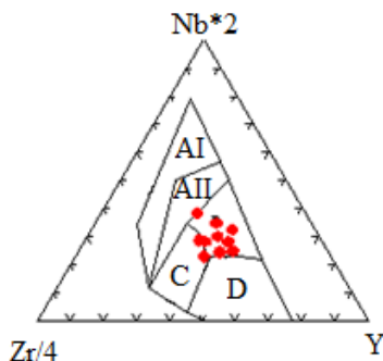
شکل ۱۱ نمودار مثلثی Nb, Y, Zr نمونه‌های مافیک و اولترامافیکی صحنه.
