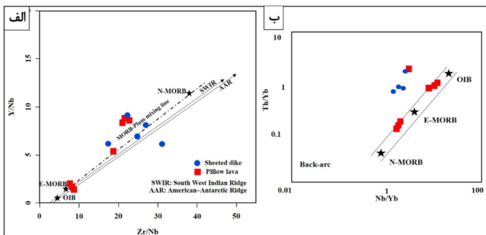
شکل ۱۳ موقعیت نمونه‌های مورد بررسی در آمیزه افیولیتی دومک بر (الف) نمودار Y/Nb نسبت به Zr/Nb و (ب) نمودار Th/Yb نسبت به Nb/Yb [۴۰]، (داده‌های E-MORB, N-MORB و OIB برگرفته از مرجع [۳۱]، داده‌های SWIR برگرفته از مرجع [۴۱] و داده‌های AAR برگرفته از مرجع [۴۲]).
