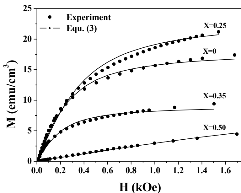
شکل ۷. برازش داده‌های تجربی M(H) با رابطه‌ی (۲) برای محاسبه‌ی مغناطش اشباعی ( M_s ) و قطر مغناطیسی ( D_m ) نانوذرات Ni_{(0.5-x)}Mn_xZn_{0.5}Fe_2O_4 . ( x = 0, 0.25, 0.35, 0.5 )
