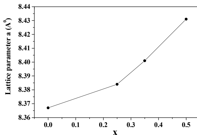
شکل ۳ تغییرات ثابت شبکه با میزان حضور منگنز (x) در نانوفریت \text{Ni}_{(0.5-x)}\text{Mn}_x\text{Zn}_{0.5}\text{Fe}_2\text{O}_4 .
