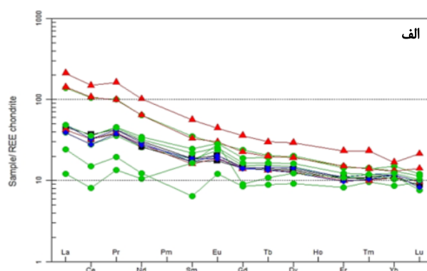
شکل ۸ الف) نمودارهای تغییرات عناصر خاکی نادر و کمیاب بهنجار شده به الف) کندریت [۲۷] و ب) NMORB [۳۱] برای آمفیبولیت‌های مورد بررسی. نشانه‌ها مشابه شکل ۵ هستند.
