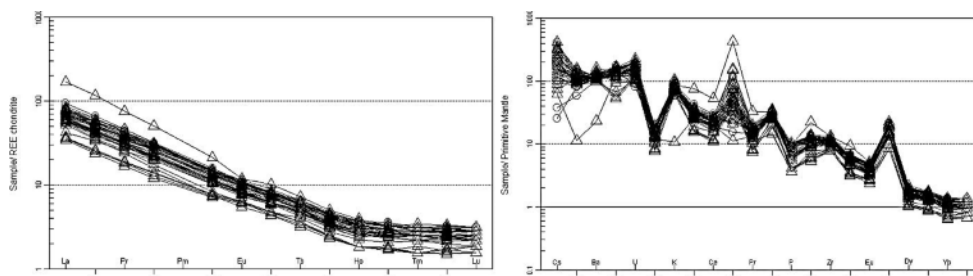
شکل ۶ نمودار عناصر نادر خاکی نرمالیز شده به کندریت [۱۵] و نمودار چند عنصری نرمالیز شده به گوشته اولیه [۱۶] برای نمونه‌های کيامکي.
