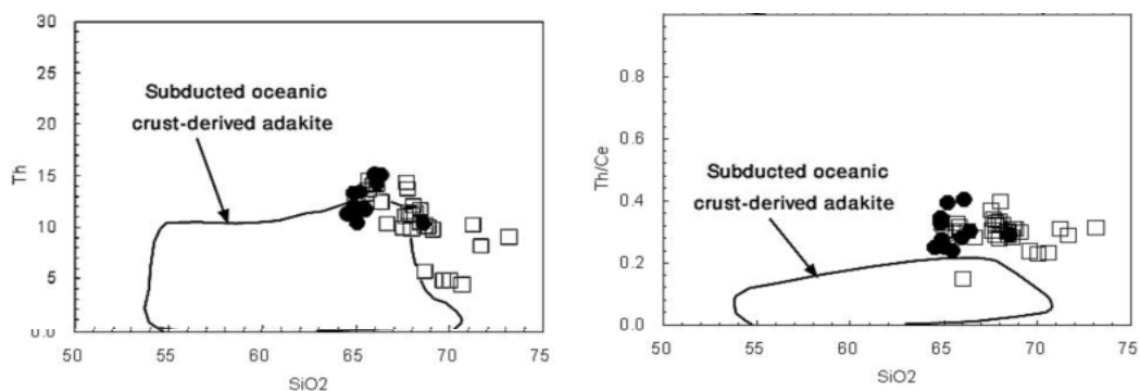
شکل ۱۱ نمودارهای SiO_2 در مقابل Th/Ce و Th . گستره مشخص شده برای آداکیت‌های حاصل از پوسته اقیانوس فرورانده شده از [۲۲]. نمادها همچون شکل ۳.
