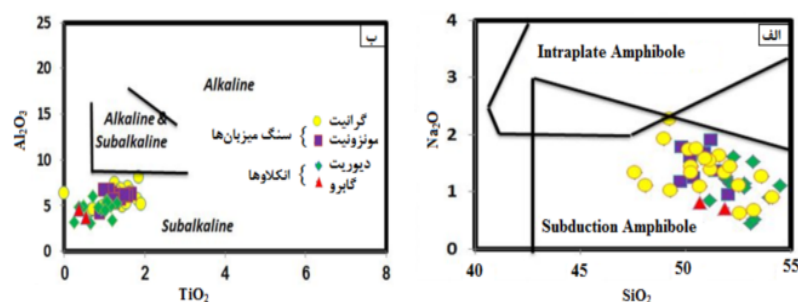
شکل ۸ الف) نمودار Na 2 O نسبت به SiO 2 بیانگر تشکیل آمفیبول‌های مورد بررسی در محیط وابسته به فروانش است [۲۷]، ب) نمودار Al 2 O 3 نسبت به TiO 2 که براساس آن، ارزیابی ماهیت سنگ‌های توده نفوذی تکیه ماهیت نیمه قلیایی دارند [۲۸].
