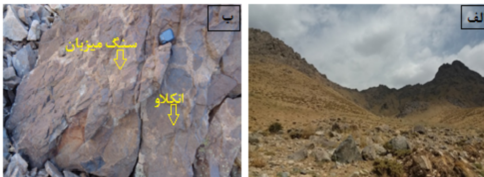
شکل ۲ روابط صحرایی میان برونوم‌ها و سنگ میزبان آن‌ها در توده نفوذی تکیه جنوب قروه: (الف) دورنمایی از منطقه مورد بررسی و (ب) فراوانی و پراکندگی برونوم دیوریتی در سنگ میزبان گرانیتی دربرگیرنده‌ی آن‌ها.
