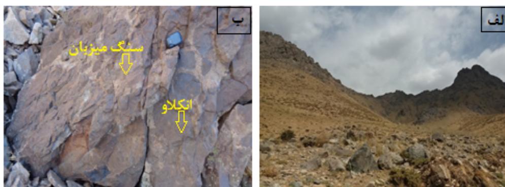
شکل ۲ روابط صحرایی میان برونوم‌ها و سنگ میزبان آن‌ها در توده نفوذی تکیه جنوب قروه: الف) دورنمایی از منطقه مورد بررسی و ب) فراوانی و پراکندگی برونوم دیوریتی در سنگ میزبان گرانیتی دربرگیرنده آن‌ها.
