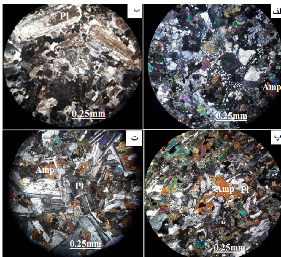
شکل ۴ تصاویر میکروسکوپی مجموعه همبندی کانیایی سازنده سنگ‌های توده نفوذی تکیه جنوب قروه (در نور قطبیده متقاطع، xpl: الف) هم‌رشدی کوارتز و ارتوکلاز (سنگ میزبان گرانیتی)، ب) بلورهای پلاژیوکلاز (سنگ میزبان مونزونیتی)، پ) بلورهای آمفیبول و پلاژیوکلاز (برونوم دیوریتی)، ت) هم‌مرز بودن بلورهای آمفیبول و پلاژیوکلاز که تعادل این دو کانی در زمان تبلور را نشان می‌دهد (برونوم گابرویی). Pl : پلاژیوکلاز، فلدسپار پتاسیم، Amp : آمفیبول.
