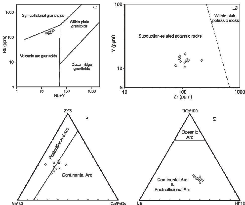
شکل ۸ الف) نمودار تغییرات Zr نسبت به Y [۳۱]؛ ب) نمودار تغییرات Rb نسبت به Nb+Y [۳۳]؛ پ) نمودار مثلثی La - TiO_2/100 - Hf*10 [۳۲]؛ ت) نمودار مثلثی Nb*50 - Zr*3 - Ce/P_2O_5 [۳۲] برای مونزونیت‌های مجموعه آذرین لار.
