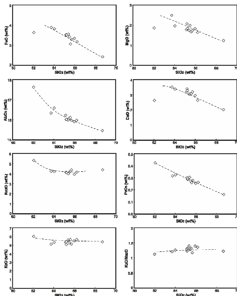
شکل ۶ نمودار تغییرات عناصر اصلی نسبت به SiO_2 برای مونزونیت‌های مجموعه آذرین لار.
