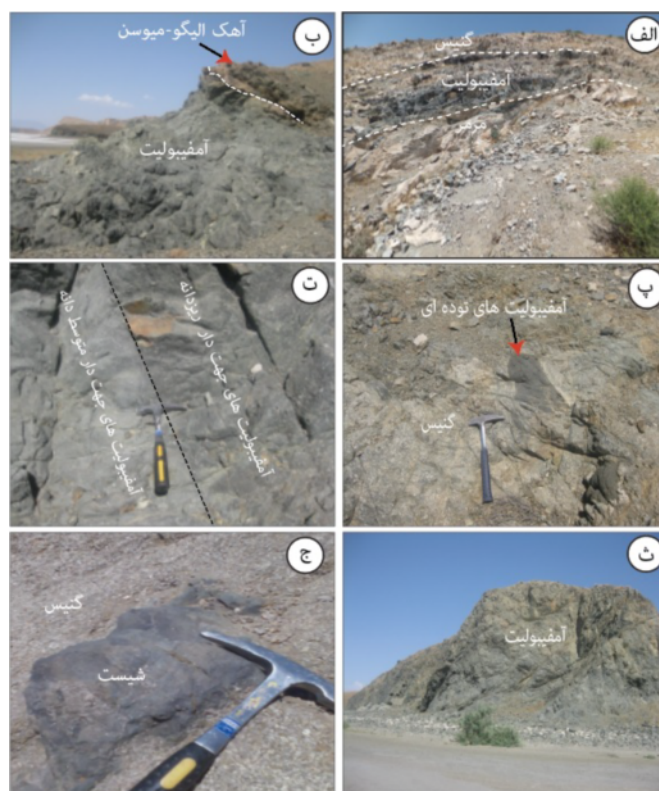
شکل ۲ الف) تناوبی از واحدهای آمفیبولیت، گنیس و آهک متبلور در ارتفاع‌های قره قشلاق (دید به سمت شمال)، ب) برخوردگاه ناپیوسته آمفیبولیت‌های منطقه با آهک‌های الیگو-میوسن، پ) قطعه‌هایی از آمفیبولیت‌های توده‌ای درون گنیس‌های منطقه (دید به سمت جنوب)، ت) آمفیبولیت‌های جهت‌یافته با دانه‌های ریز و متوسط (دید به سمت جنوب شرق)، ث) رخنمون آمفیبولیت در ساحل غربی دریاچه ارومیه (دید به سمت جنوب) و ج) برخوردگاه شیست سبز توده‌ای با گنیس (دید به سمت شمال - شمال شرق).
