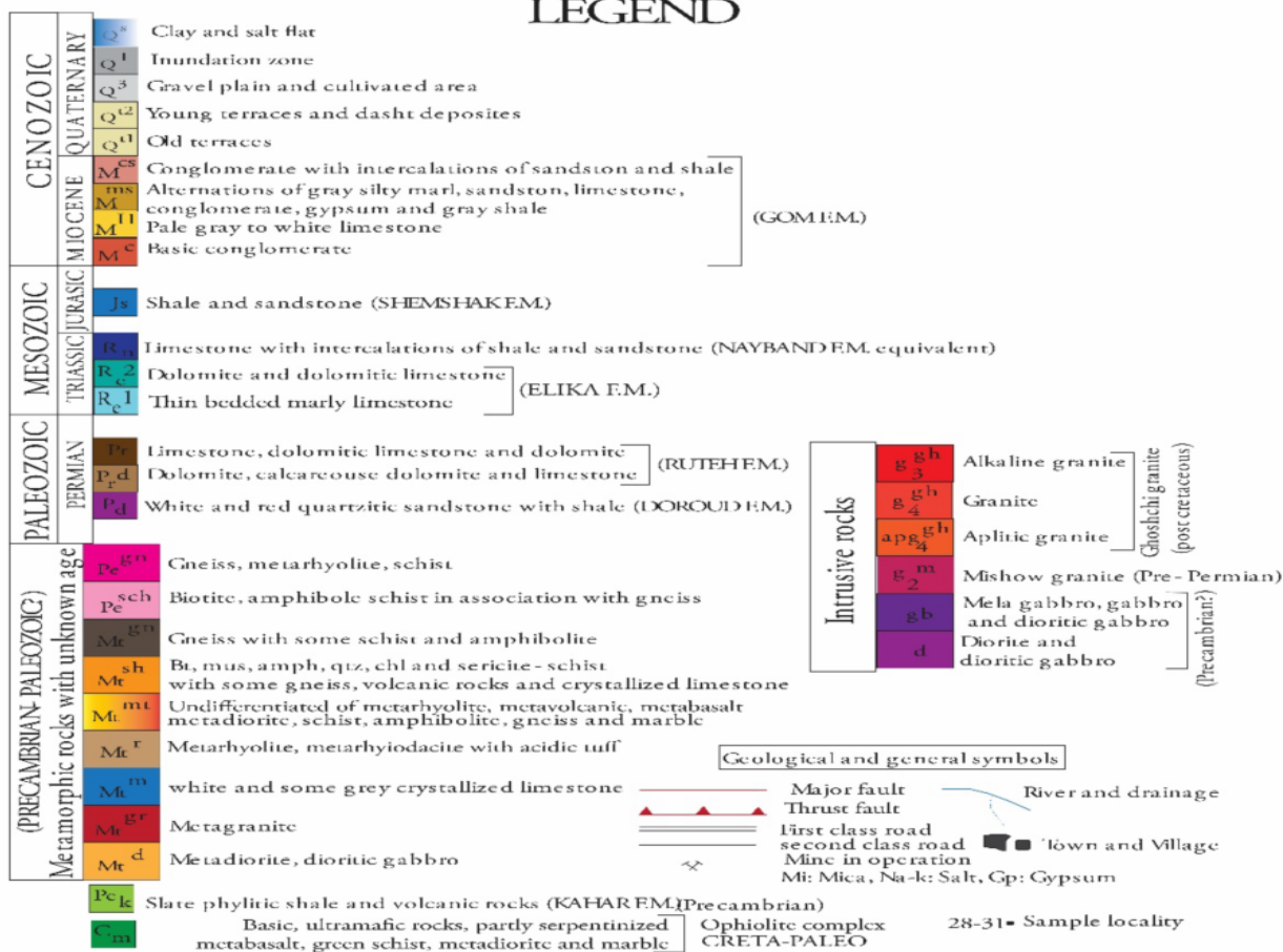
شکل ۱ نقشه زمین‌شناسی منطقه مورد بررسی، برگرفته از نقشه‌های زمین‌شناسی ۱:۱۰۰۰۰۰ [۵] و سلماس [۶].
