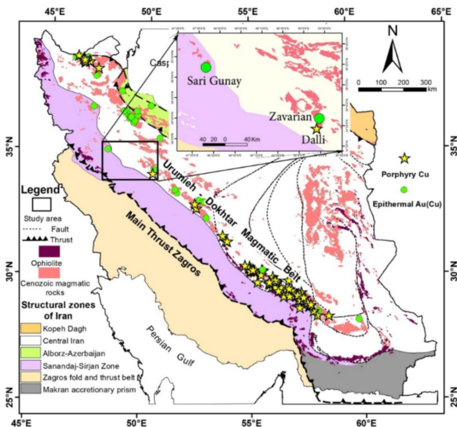
شکل ۱ موقعیت جغرافیایی کانسار زواریان (کمان ماگمایی ارومیه-دختر و کانسار ساری گونای پهنه ساندج-سیرجان، برگرفته از نقشه زمین شناسی ایران با مقیاس ۱:۱۰۰۰۰۰۰، سازمان زمین شناسی و اکتشافات معدنی کشور، ۱۳۸۵).
