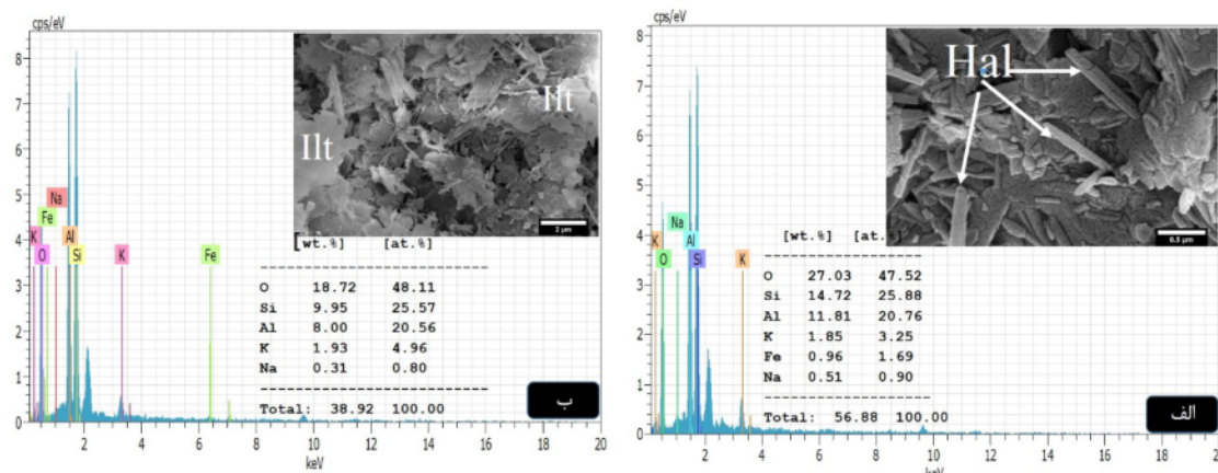
شکل ۶ تصاویر میکروسکوپ الکترونی روبشی اثر میدانی (FE-SEM) به همراه طیف‌های تجزیه نقطه‌ای EDS. الف) بلورهای لوله‌ای شکل هالوئیزیت در زمینه‌ای از بلورهای تخته‌ای هالوئیزیت. با بزرگنمایی ۱۲۰۰۰ برابر و ب) بلورهای ورقه‌ای کوچک ایلیت با بزرگنمایی ۶۰۰۰۰ برابر (Ht: ایلیت و Hal: هالوئیزیت).
