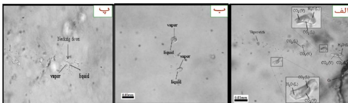
شکل ۶ انواع سیال‌های درگیر دیده شده در نمونه‌های کوارتز منطقه مورد بررسی: الف) سه فازی ( \text{H}_2\text{O}-\text{CO}_2-\text{NaCl} ) ب) دو فازی ( \text{LCO}_2 + \text{VCO}_2 + \text{LH}_2\text{O} ) پ) پدیده دم بریدگی.
