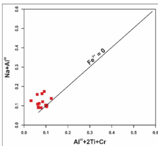
شکل ۷ نمودار Al^{VI}+2Ti+Cr نسبت به Na+Al^{IV} [۵۰] برای تعیین گریزندگی اکسیژن ماگمای مادر بازالت‌های گزبلند.
