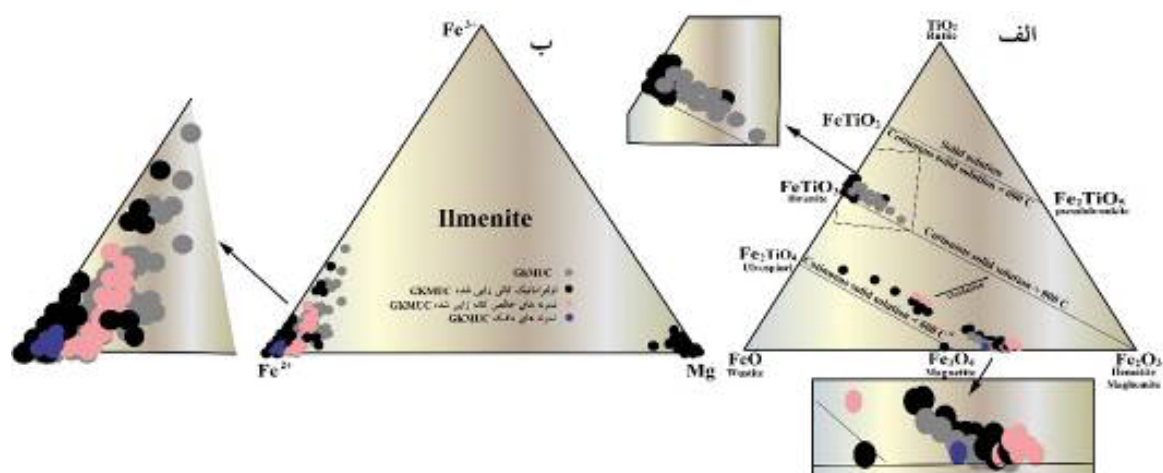
شکل ۸ الف) نمودار سه تایی سامانه جامد \text{TiO}_2\text{-FeO-Fe}_2\text{O}_3 که خطوط اتصالیه انحلال جامد بین مگنتیت و تیتانومگنتیت را نشان می‌دهد [۱۸]، ب) نمودار مثلثی \text{Mg-Fe}^{2+}\text{-Fe}^{3+} ، [۲۲، ۲۱]، و موقعیت اکسیدهای Fe-Ti در آن که ایلمنیت ها در فرامافیک‌های کانه‌زایی شده هم با MgO بالا و هم با MgO پایین ولی در بقیه انواع سنگ‌های هر دو توده از نوع MgO پایین هستند.
