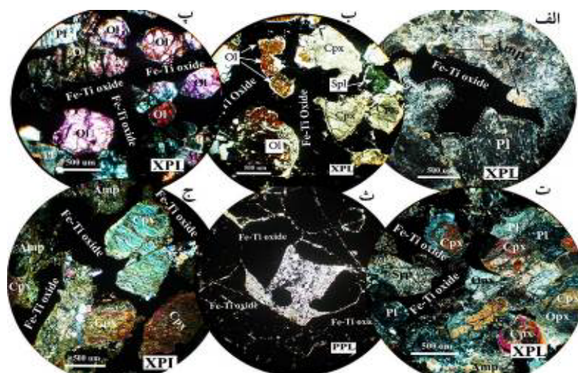
شکل ۴ تصاویر میکروسکوپی از سنگ‌های GKMUC: الف) آنورتوزیت کانی‌زایی شده، ب) نمونه ورلیت کانه زایی شده، پ) نمونه‌های دونیت پلاژیوکلازدار کانه‌زایی شده، ت) نمونه گابروی کانی‌زایی شده دارای ارتوپيروكسن، ث) انباشت سنگ خالص اکسید Fe-Ti، و ج) نمونه پیروکسنیت کانه زایی شده. نشانه‌های اختصاری مانند شکل ۳ است.
