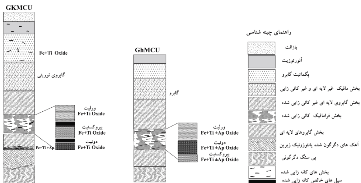
شکل ۹ مقایسه ستون‌های چینه‌نگاری توزیع واحدهای سنگی و کانه‌زایی کانه اکسید Fe-Ti در توده‌های GhCUM و GKCUM.
