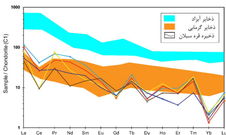
شکل ۱۰ الگوی توزیع عناصر خاکی نادر به‌نحار شده نسبت به کندریت C1 [۳۹] برای نمونه‌های کانسنگ قره سبلان در مقایسه با ذخایر منگنز مختلف آبراد [۴۰] و گرمابی [۶].
