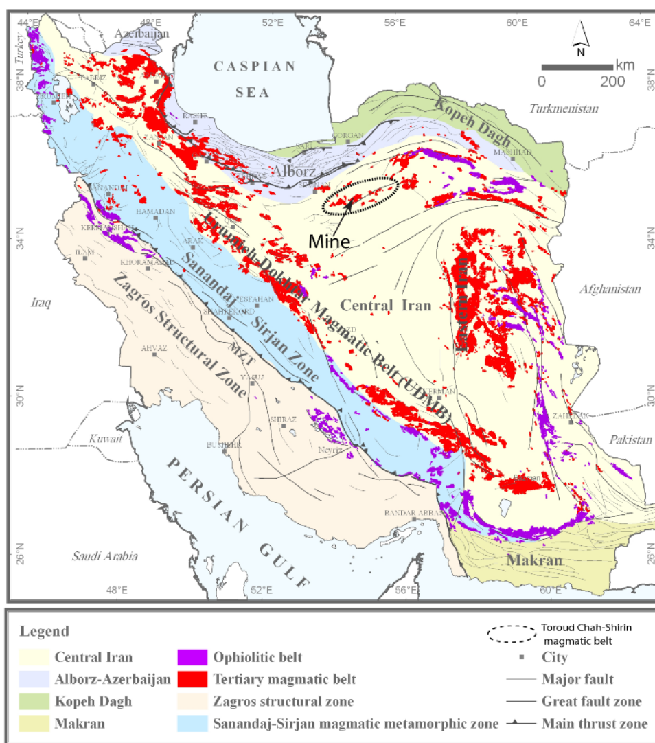
شکل ۱ موقعیت منطقه مورد بررسی و معدن فیروزه- طلای دامغان (علامت پیکان) و کمان آتشفشانی- نفوذی تروود چاه شیرین (منحنی خط چین) در نقشه فعالیت ماگمایی ایران برگرفته از مرجع [۱] با تغییرات جزئی.
