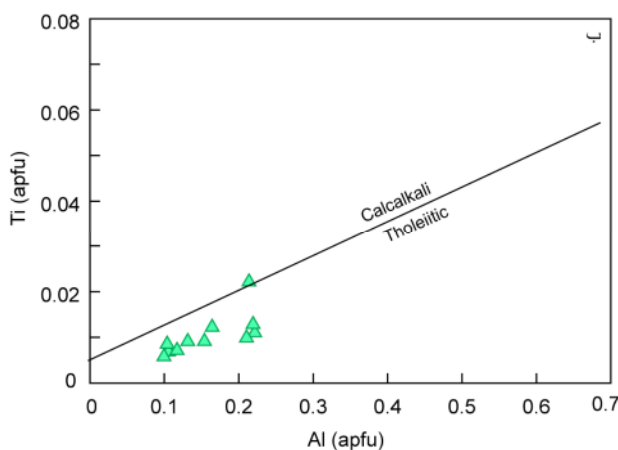
شکل ۷ نمودارهای الف) Ti نسبت به Ca+Na و ب) Ti نسبت به Al برای تشخیص ماهیت کلینوپیروکسن بازالت های متاع [۸].
