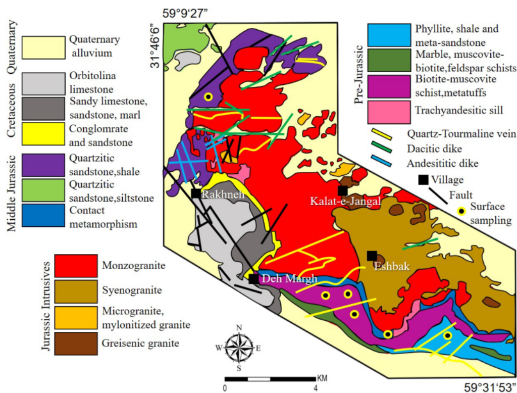
شکل ۲ نقشه زمین‌شناسی ساده شده منطقه شاهکوه همراه با واحدهای سنگی رخنمون‌یافته در منطقه [۱۰].
