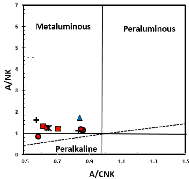
شکل ۶ موقعیت نمونه‌های سنگی حصاروئیه بر روی نمودار شاخص آلومینیوم [۱۱]، نمونه‌ها در محدوده مت‌آلومین قرار می‌گیرند A/NK: Al_2O_3 / (Na_2O + K_2O) , A/CNK: Al_2O_3 / (CaO + Na_2O + K_2O) ، نشانه‌ها مشابه شکل ۴ می‌باشد.
