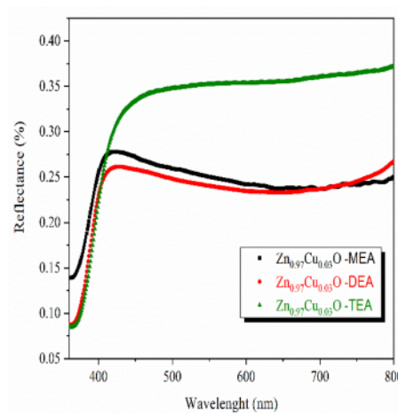
شکل ۸. الف) طیف بازتاب پخشی و ب) نمودار تعیین گاف نوری نانوذرات Zn_{0.97}Cu_{0.03}O تهیه‌شده با پایدارسازهای مونو- دی - و تری- اتانول آمین.
