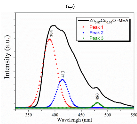
شکل ۹. الف) طیف نورتایی نانوذرات Zn_{0.97}Cu_{0.03}O تهیه‌شده با پایدارسازهای آمینوالکلی، ب) برازش گاوسی قله‌های نورتایی نانوذرات Zn_{0.97}Cu_{0.03}O تهیه‌شده با پایدارساز مونو اتانول آمین.
