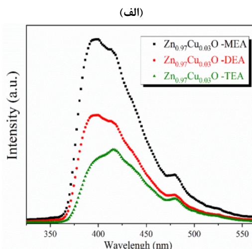
شکل ۹. الف) طیف نورتایی نانوذرات Zn_{0.97}Cu_{0.03}O تهیه‌شده با پایدارسازهای آمینوالکلی، ب) برازش گاوسی قله‌های نورتایی نانوذرات Zn_{0.97}Cu_{0.03}O تهیه‌شده با پایدارساز مونو اتانول آمین.
