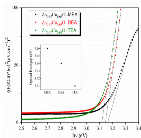
شکل ۸. الف) طیف بازتاب پخشی و ب) نمودار تعیین گاف نوری نانوذرات Zn_{0.97}Cu_{0.03}O تهیه‌شده با پایدارسازهای مونو- دی - و تری- اتانول آمین.
