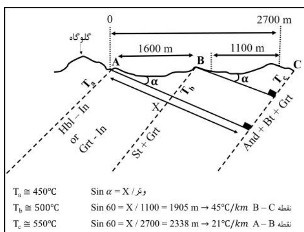
شکل ۱۶ شب (مبنی بر مایه) محاسبه شده در بخش غربی مجموعه دگرگونه دهسلم (منطقه گلوگاه).
