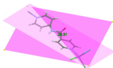
شکل ۶ نمایش صفحه‌های دربردارنده حلقه‌های ایزونیکوتینیل و پیریدیل.
