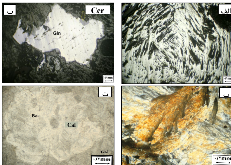
شکل ۴ تصاویر میکروسکوپی از الف) گالن با رخ شمشیری (XPL)، ب) تبدیل گالن (Gln) در لیه‌ها به سروزیت (Cer)، پ) باریت با بافت پرماند و ماکل تکراری (XPL) و ت) حضور باریت (Ba) در زمینه کلسیت (Cal) (PPL). (نشانه‌های اختصاری بر گرفته از مرجع [۲۵] هستند).
