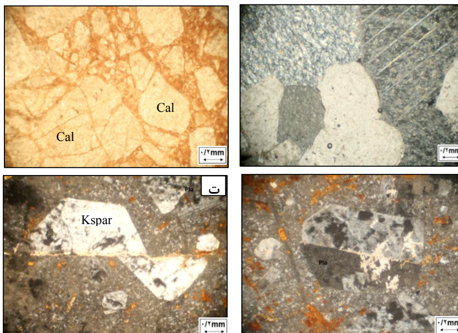
شکل ۲ تصاویر میکروسکوپی از الف- بلورهای کلسیت (Cal) به همراه رخ لوزی شکل و بافت موزاییکی (در نور قطبیده متقاطع، XPL). ب- سنگ آهک برشی که توسط اکسید آهن سیمانی شده است (در نور قطبیده صفحه‌ای، PPL)، پ- تصویری از واحد مونزونیتی با بافت پورفیری (XPL) و ت- بلور شکسته شده فلدسپار قلیایی (Ksp) که محل شکستگی با کربنات پر شده است (XPL). (نشانه‌های اختصاری برگرفته از مرجع [۲۵] هستند).
