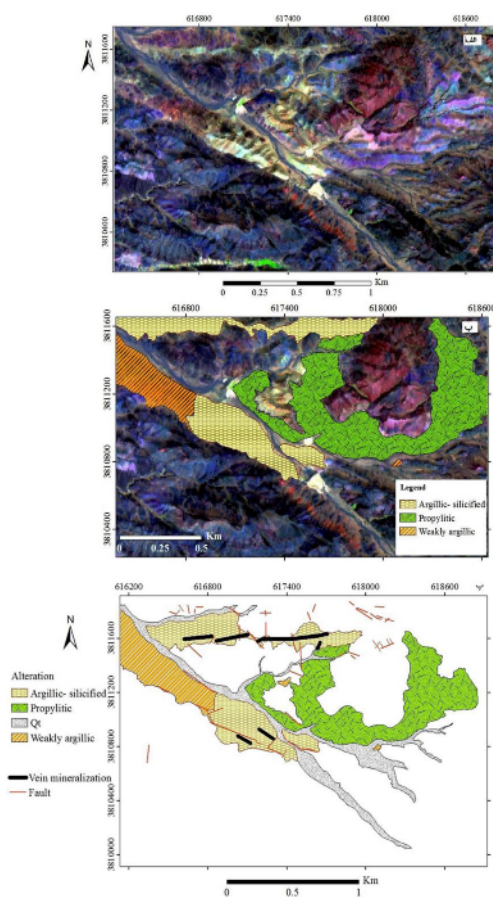
شکل ۴ الف) تصویر ماهواره‌ای پردازش‌شده از منطقه مورد بررسی که روند خطی دگرسانی آرژیلی-سیلیسی (به ویژه در شمال منطقه) مشهود است، ب) تطبیق نقشه دگرسانی بر تصویر ماهواره‌ای و پ) نقشه دگرسانی و کانی‌سازی در منطقه بیدوک.
