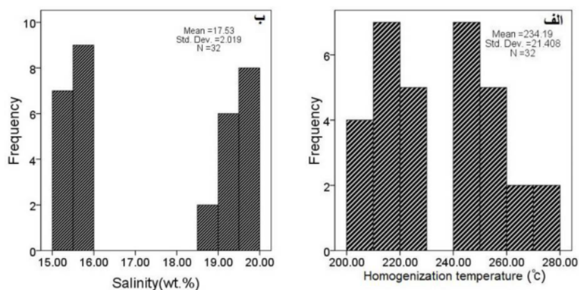
شکل ۱۰ توزیع الف) دمای همگن‌شدگی و ب) شوری سیال‌ها در رگه‌های طلا دار بیدوک.
