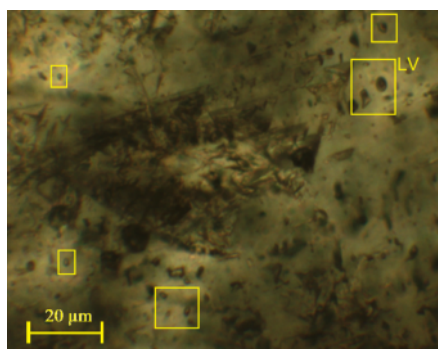
شکل ۹ تصویر میکروسکوپی از سیال‌های درگیر دوفازی (LV) درون کانی کوارتز در منطقه بیدوک.
