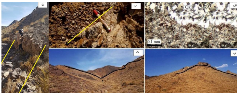
شکل ۵ الف) مقطعی از رگه سیلیسی که در لبه به کانی‌های رسی دگرسان شده است (نور XPL). و ب) دگرسانی آرژیلی در لبه رگه سیلیسی-اکسید آهن، پ و ت) رخنمون رگه‌های سیلیسی-اکسیدآهنی با روند شمال‌غرب-جنوب‌شرقی در منطقه بیدوک (دید به سمت شرق)، ث) راستای رگه سیلیسی (خطوط زرد) منطبق بر سطح گسل که در کف آبراهه رخنمون یافته است. (دید عکس به سمت شمال). (Qtz): کوارتز [۱۵]
