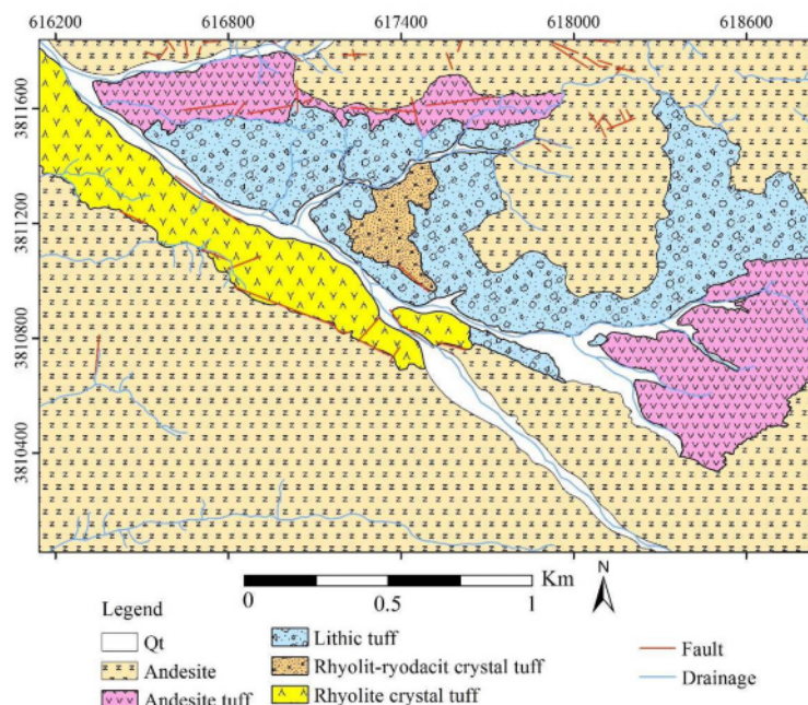
شکل ۳ نقشه زمین‌شناسی منطقه بیدوک.
