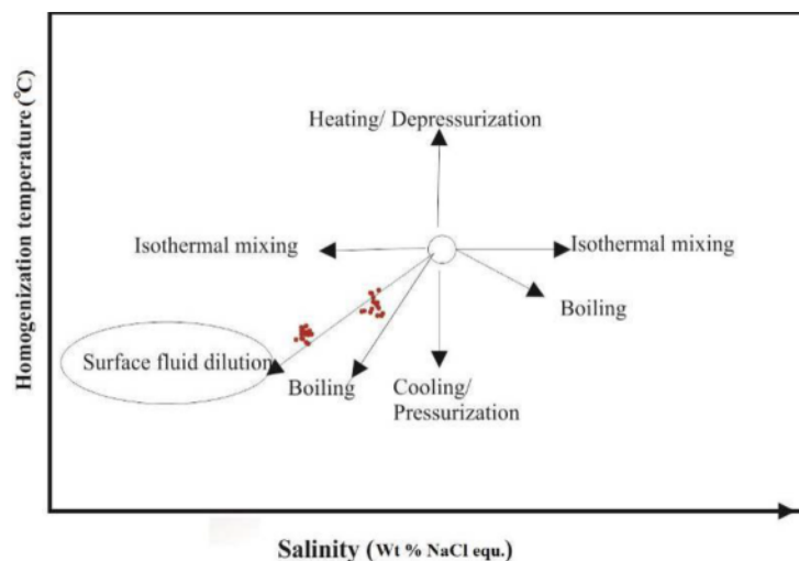
شکل ۱۲ نمودار دمای همگن‌شدگی به شوری سیال‌های درگیر که رقیق‌شدگی توسط سیال‌های سطحی مهم‌ترین عامل موثر در روند ته‌نشینی کوارتز در منطقه بیدوک بوده است [۳۷]. جدول ۴ مقایسه ویژگی‌های مختلف رگه کوارتز-سولفید بیدوک با تعدادی از کانسارهای طلای رگه‌ای اپی‌ترمال در ایران و سایر نقاط جهان.
