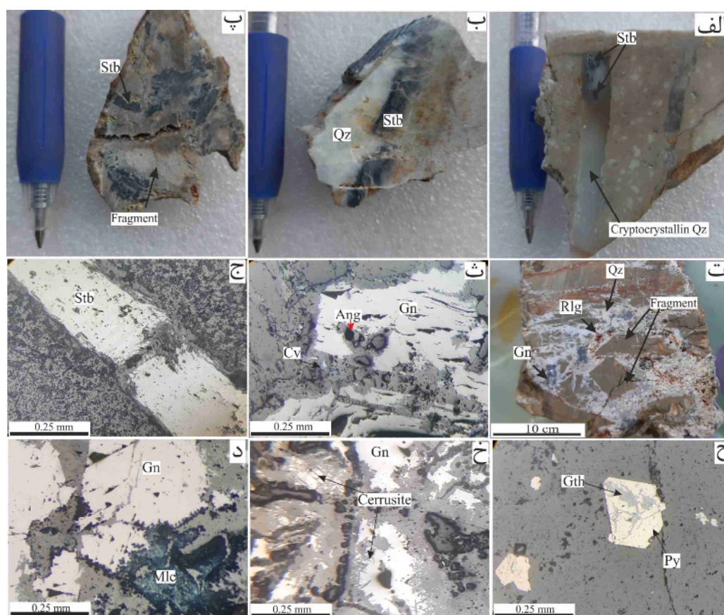
شکل ۴ نمونه دستی از کانی‌سازی در منطقه کوه شورو و تصاویر میکروسکوپی در نور بازتابی از الف) رگچه‌های کوارتز نهان بلوری-استیبینیت در واحد داسیتی، ب) رگه کوارتز-استیبینیت در واحد داسیتی، پ) استیبینیت-کوارتز نهان بلوری در برش گسلی با قطعه‌هایی از سنگ میزبان داسیتی. ت) گالن-زرنیخ قرمز-کوارتز در برش گسلی با قطعه‌هایی از واحد شیلی، ث) گالن از لبه در حال تبدیل به آنگلیت (PPL)، ج) ستون‌های کشیده استیبینیت (PPL)، ح) پیریت بیشتر به صورت شکل‌دار تا نیمه شکل‌دار در حال تبدیل به گوتیت (PPL)، خ) تبدیل گالن به سروزیت (PPL)، د) مالاکیت (PPL). پیریت = Py، استیبینیت = St، آنگلیت = Ang، گوتیت = Gth، کوولیت = Cv، گالن = Gn، زرنیخ قرمز، Qz = کوارتز و Mlc = مالاکیت [۱۳].
