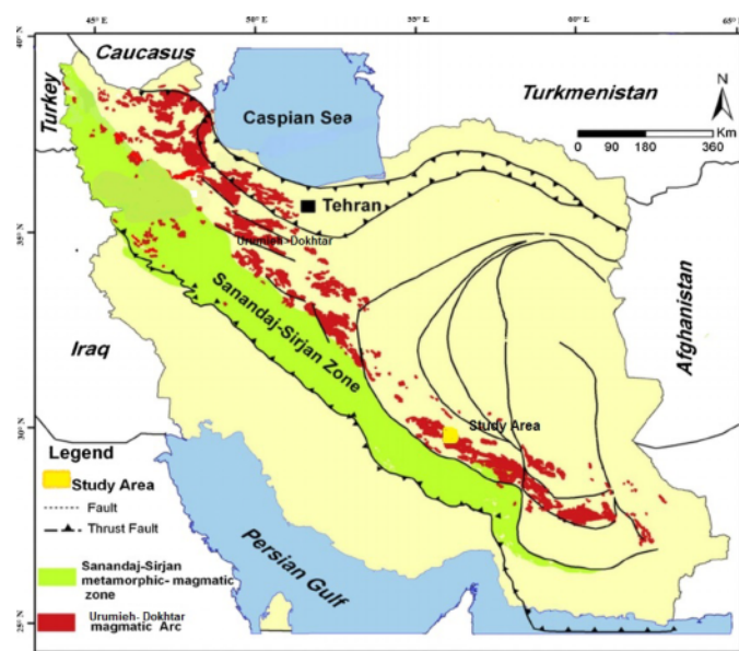
شکل ۲ موقعیت منطقه مورد بررسی در پهنه ساختاری ارومیه دختر [۲].
