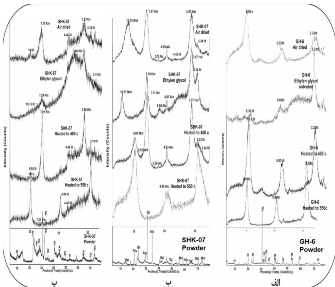
شکل ۷ الگوهای XRD نمونه‌های کائولن با تیمارهای مختلف: الف) نمونه GH-6، ب) نمونه SHK-07 و پ) نمونه SHK-57. نشانه‌های اختصاری به کار رفته (rs): جارسیت، Ms: مسکویت، Illt: ایلیت، Qz: کوارتز، Gp: ژپیس، Hal: هالوزیت، Alu: آلونیت، Mnt: مونت‌موریلونیت، Kln: کائولینیت و Ab: آلبیت) برگرفته از مرجع [۵] هستند.
