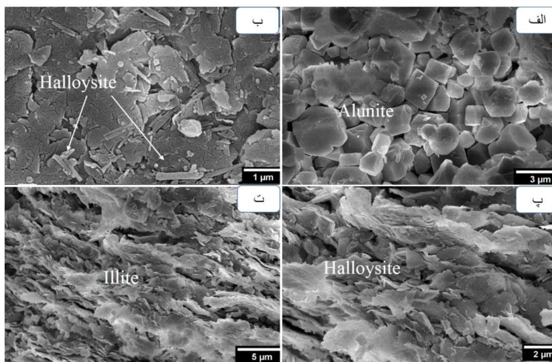
شکل ۹ تصاویر میکروسکوپ الکترونی روبشی اثر میدانی از الف) بلورهای خود شکل و مکعبی آلونیت، بزرگنمایی ۱۵۰۰۰ برابر. ب) بلورهای تخته-ای هالوئیزیت، بزرگنمایی ۶۰۰۰۰ برابر. پ) بلورهای لوله‌ای شکل هالوئیزیت در زمینه‌ای از بلورهای تخته‌ای شکل هالوئیزیت، بزرگنمایی ۱۰۰۰۰۰ برابر و ت) بلورهای ورقه‌ای کوچک با لبه‌های منحنی ایلیت، بزرگنمایی ۲۵۰۰۰ برابر.
