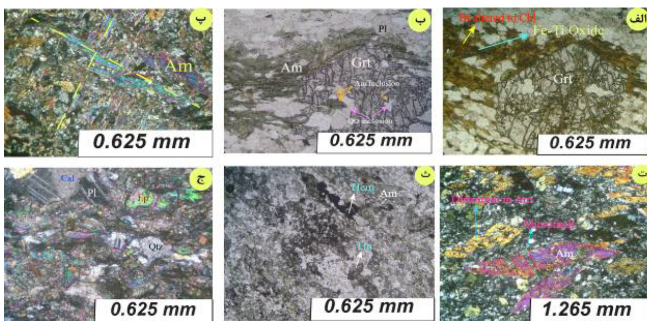
شکل ۳ الف) همزیستی گارنت و بیوتیت که بیوتیت در فاز پسرودگی به کلریت تجزیه شده است. اکسیدهای Fe-Ti دار در راستای رخ ها و لبه های بیوتیت آزاد شده اند. گارنت دارای شکستگی های لانه زنبوری و نیز پسا زمین ساخت است. ب) همزیستی گارنت و آمفیبول کلسیمی که میانبارهای کوارتز دارای بقایایی از آمفیبول هستند. آمفیبولیت بدون گارنت شامل: پ) دو دسته آمفیبول که به صورت متقاطع و نسبت به هم تصادفی قرار گرفته اند. ت) اعوجاج و ریزگسل در آمفیبول. ث) تیتانیت و هماتیت در کنار آمفیبول. ج) شست های اپیدوت-دار که پلاژیوکلاز با ماکل دگرشکلی، کلسیت و اپیدوت در آن مشخص است.
