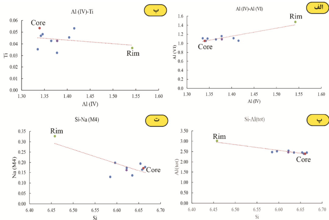
شکل ۵ نمودارهای Al(IV) – Al(VI) و Ti-Al(IV) (الف و ب) منطقه‌بندی شیمیایی در آمفیبول از مرکز به لبه را نشان می‌دهند. پ و ت) نمودارهای Si-Al(tot), Si-Na(M4) که براساس آنها با افزایش Al tot و Na (M4) مقدار Si کاهش می‌یابد (مقادیر برحسب apfu است).
