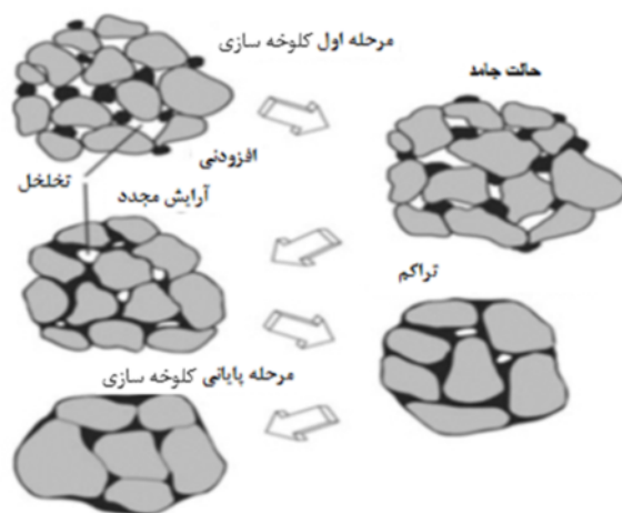
شکل ۲ سازوکار کلوخه‌سازی \text{SiC} در حضور فاز مایع.
