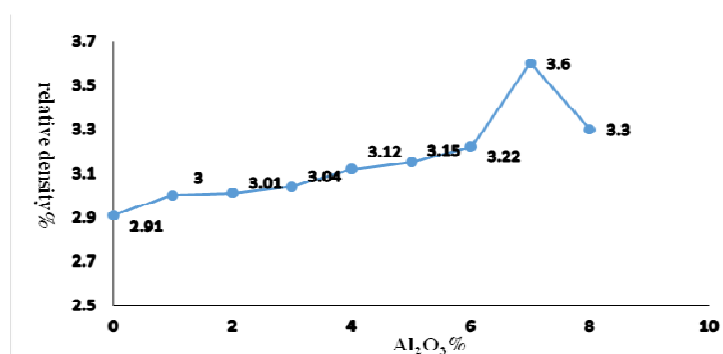
شکل ۳ چگالی نمونه‌ها نسبت به مقدار آلومینا.
