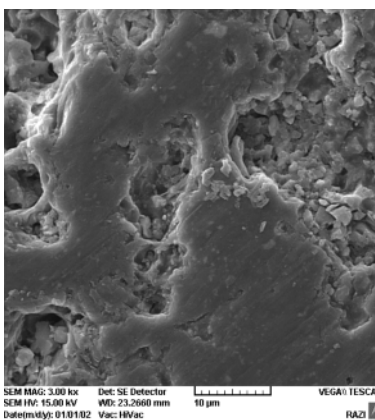
شکل ۶ تصویر SEM نمونه کلوخه سازی شده SiC دربردارنده ۸ درصد وزنی Al_2O_3 .
