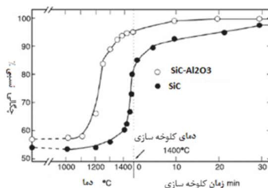
شکل ۴ مقایسه چگالی نسبی نمونه های با و بدون Al_2O_3 نسبت به زمان کلوخه سازی.
