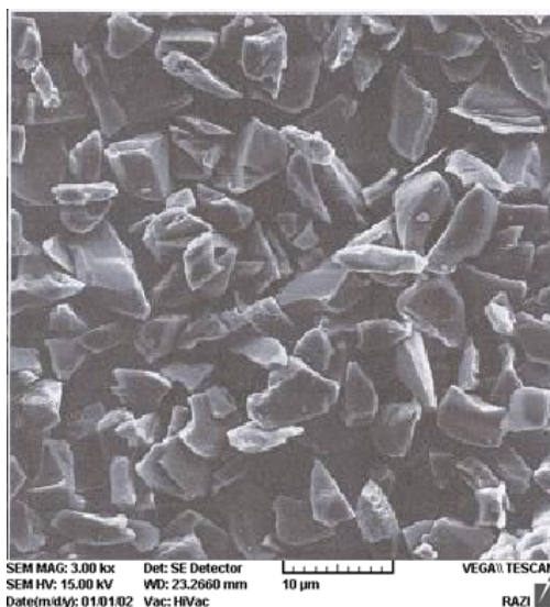
شکل ۱ تصویر SEM از پودر SiC-Al_2O_3 آسیاب شده.
