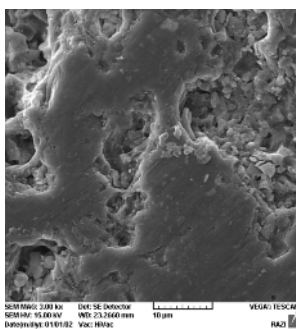
شکل ۶ تصویر SEM نمونه کلوخه سازی شده \text{SiC} دربردارنده ۸ درصد وزنی \text{Al}_2\text{O}_3 .
