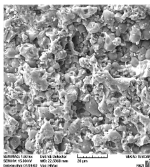
شکل ۵ تصویر SEM از نمونه \text{SiC} کلوخه سازی شده در دمای ۱۴۰۰ درجه سانتیگراد.
