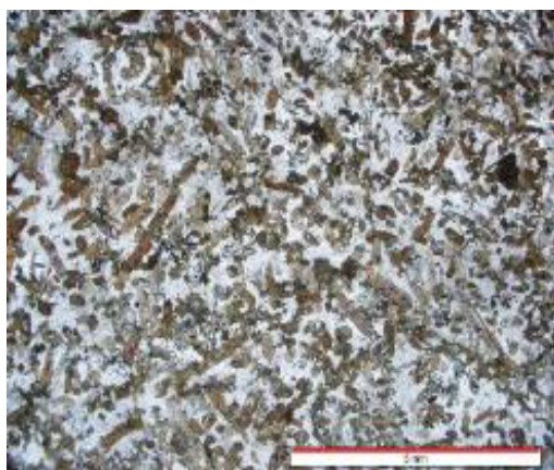
شکل ۴ تصاویر میکروسکوپی از سنگ‌های سازنده بخش‌های لبه‌ای توده و حضور هورنبلندهای قهوه‌ای کوچک سوزنی شکل و پلاژیوکلاز و کمی پیروکسن در گابرو دیوریت‌های دانه‌ریز منطقه پلنگ‌در. (تصاویر سمت راست و چپ به ترتیب در نور XPL و PPL، ثبت شده‌اند).
