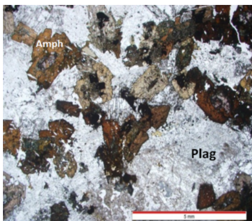
شکل ۵ تصاویر میکروسکوپی از گابروهای پگماتوئیدی بسیار دانه‌درشت. حضور پلاژیوکلاز با ماکل چندریخت همراه با میانبارهایی از هورنبلند قهوه‌ای، پیروکسن و آپاتیت قابل توجه هستند. بلورهای آپاتیت به صورت چند تیغه کوچک با رنگ خاکستری روشن درون هورنبلند قهوه‌ای به روشنی دیده می‌شوند. (تصاویر سمت راست و چپ به ترتیب در نور XPL و PPL، ثبت شده‌اند).
