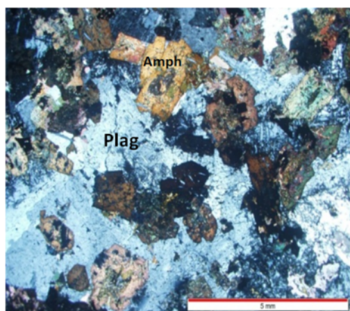
شکل ۵ تصاویر میکروسکوپی از گابروهای پگماتوئیدی بسیار دانه‌درشت. حضور پلاژیوکلاز با ماکل چندریخت همراه با میانبارهایی از هورنبلند قهوه‌ای، پیروکسن و آپاتیت قابل توجه هستند. بلورهای آپاتیت به صورت چند تیغه کوچک با رنگ خاکستری روشن درون هورنبلند قهوه‌ای به روشنی دیده می‌شوند. (تصاویر سمت راست و چپ به ترتیب در نور XPL و PPL، ثبت شده‌اند).
