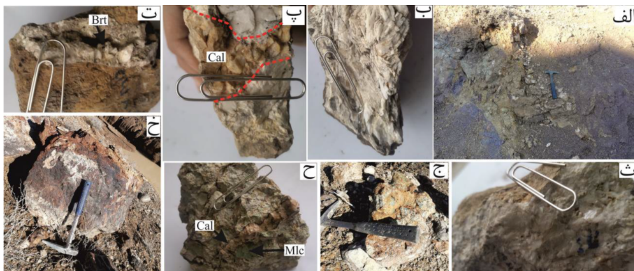
شکل ۵ تصاویر صحرایی و نمونه دستی از کانی‌سازی منطقه اکتشافی باریت مشکان. الف) رخنمون رگه باریت در صحرا، ب) باریت با بافت صفحه-ای، پ) باریت با بافت صفحه‌ای که توسط رگه کلسیتی قطع شده، ت) باریت با بافت شعاعی، ث) باریت با بافت توده‌ای، ج) آزوریت همراه با اکسید آهن در واحد کنگلومرای، ح) کانی‌سازی مالاکیت در واحد کنگلومرای که توسط رگچه کلسیتی قطع شده است، خ) اکسیدهای آهن (هماتیت و گوتیت). اختصارات: Cal = کلسیت، Brt = باریت، Mlc = مالاکیت [۱۴].
