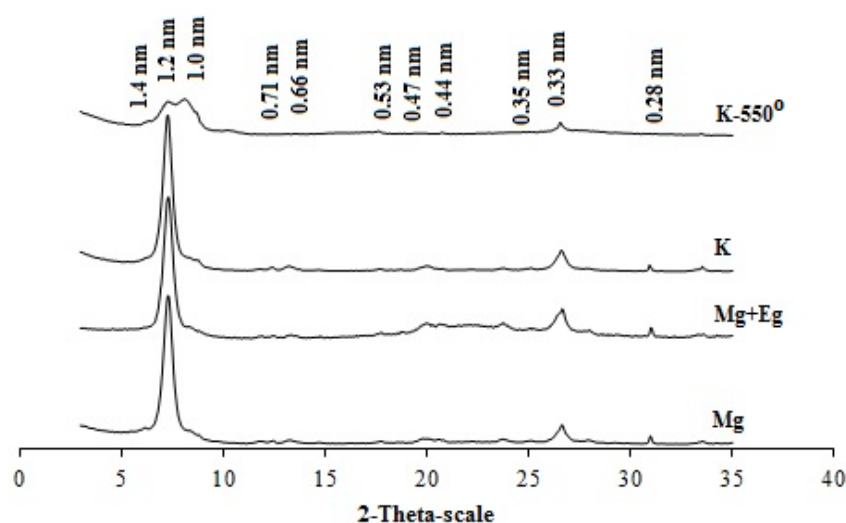
شکل ۱ پراش نگاشت‌های پرتوی ایکس رس نمونه شاهد. (Mg نمونه اشباع با منیزیم، Mg-Eg: نمونه اشباع با منیزیم و اتیلن گلیکول، K: نمونه اشباع با پتاسیم و K-550: نمونه اشباع با پتاسیم و گرمادهی شده تا ۵۵۰ درجه سانتی‌گراد).
