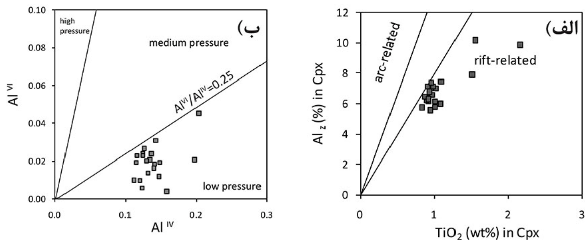
شکل ۸ الف) نمودار \text{TiO}_2 نسبت به \text{Al}_2 برای تعیین محیط زمین‌ساختی تشکیل بازالت‌های مورد بررسی در منطقه گشت-ماسوله براساس شیمی کلینوپیروکسن [۴۴] و ب) نمودار \text{Al}^{\text{IV}} نسبت به \text{Al}^{\text{VI}} برای تعیین گستره فشار تبلور کانی کلینوپیروکسن از ماگمای مادر سنگ‌های بازالتی گشت-ماسوله [۲۹].
