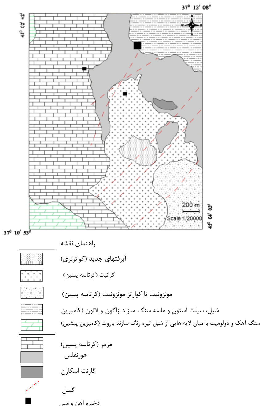
شکل ۲ نقشه ساده شده زمین‌شناسی منطقه آغبالاغ اشنویه (برگرفته از مرجع [۱۲] با تغییرات).
