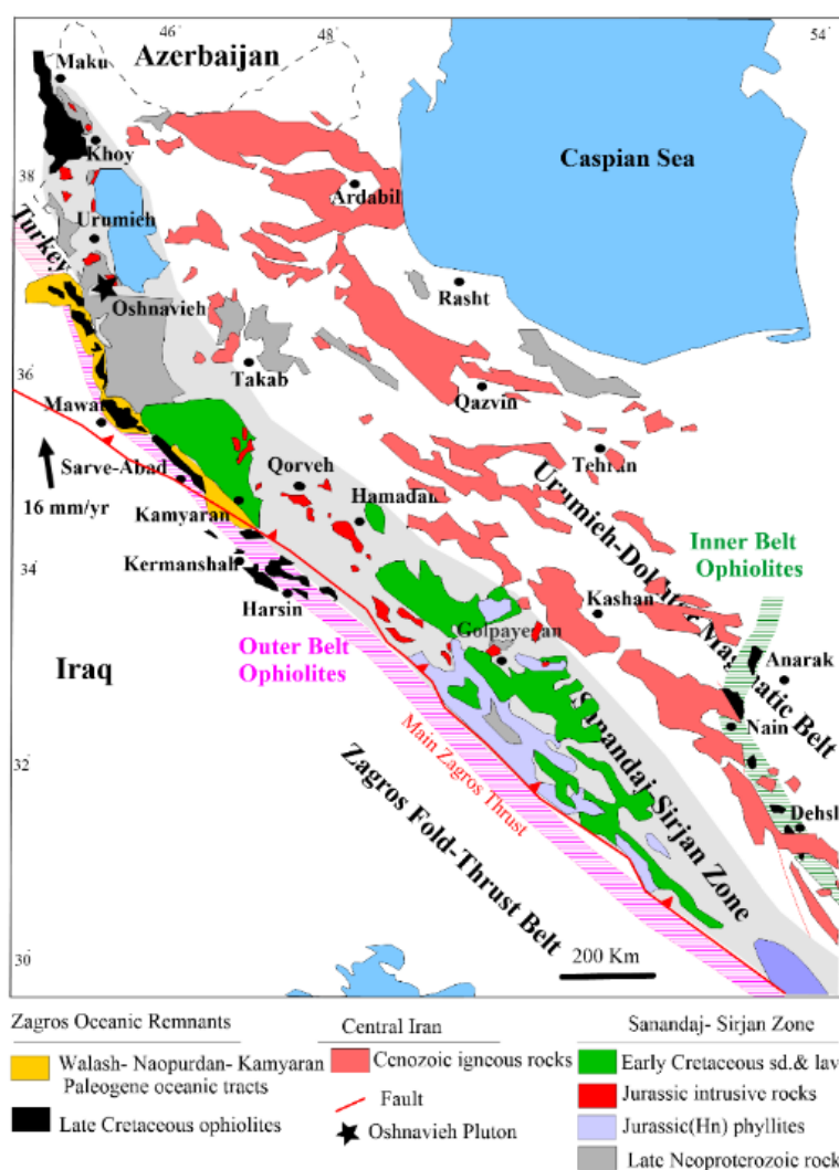
شکل ۱ نقشه بخشی از پهنه ساختاری ایران (بر گرفته از مرجع [۸] با تغییرات) که در آن جایگاه منطقه آغلایغ با علامت ستاره نشان داده شده است.
