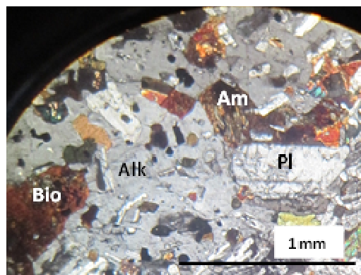
شکل ۱۰ بافت پوئیکلیتیک در گرانیت منطقه‌ی لاله‌زار. کانی‌های ریزپلاژیوکلاز، آمفیبول و بیوتیت به‌صورت ادخال درون فلدسپار قلیایی قرار دارند.
