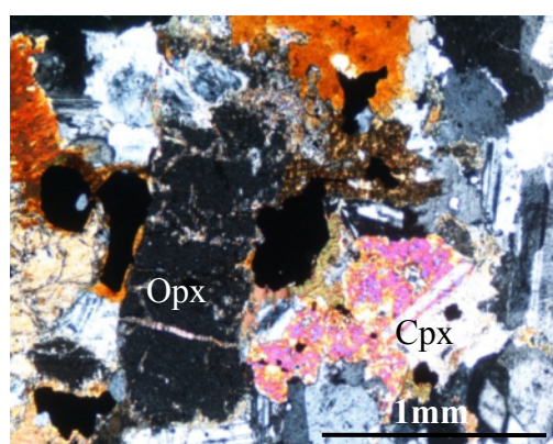
شکل ۱۲ کلینوپیروکسن و ارتوپیروکسن در گابرویدوریت منطقه.
