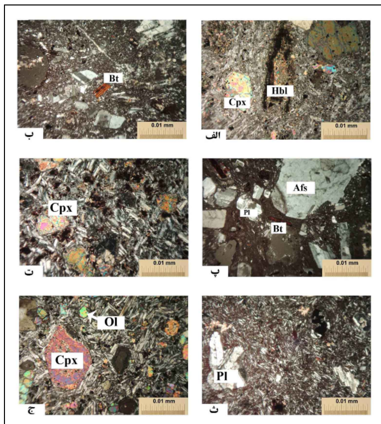
شکل ۳ تصاویر میکروسکوپی از مقاطع نازک (نور XPL) (الف) هورنبلند پیروکسن آندزیت، (ب) بیوتیت آندزیت، (پ) بیوتیت هیالوآندزیت، (ت) پیروکسن آندزیت، (ث) آندزیت، (ج) الیوین بازالت، (د) پلاژیوکلاز، (ه) کلینوپیروکسن، (و) آفس: فلدسپات قلیایی، (ز) بیوتیت، (ح) الیوین، (ط) هورنبلند [۱۷].
