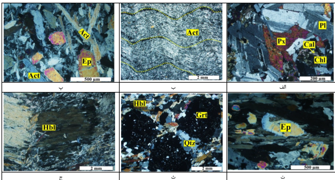
شکل ۴ تصاویری میکروسکوپی از ویژگی‌های بارز متابازیت‌های مجموعه دگرگونی-آذرین جنوب دوچاه (در نور قطبیده متقاطع، XPL): الف- گابرودیوریت اولیه به عنوان سنگ مادر بخشی از متابازیت‌ها، ب- اکتینولیت شیست و چین‌های نمایان آن، پ- اپیدوت اکتینولیت شیست، ت- ریزساختار اپیدوت‌ماهی در اپیدوت اکتینولیت شیست، ث- گارنت آمفیبولیت و ج - ریزدانه شدن هورنبلند در آمفیبولیت. (علائم اختصاری کانی‌ها عبارتند از: Pl: پلاژیوکلاز، Ep: اپیدوت، Px: پیروکسن، Hb: هورنبلند، Ac: اکتینولیت و Gt: گارنت).
