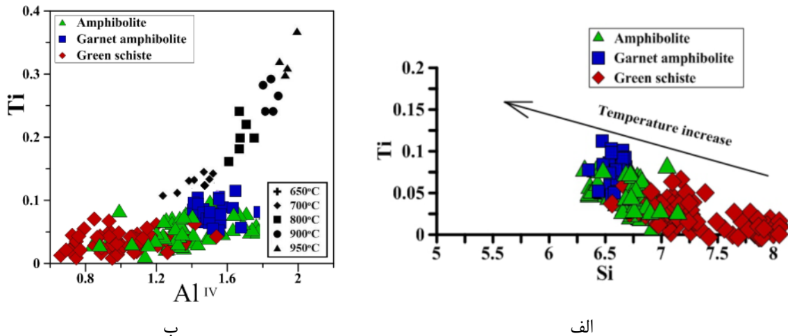
شکل ۸ موقعیت ترکیبی آمفیبول‌های متابازیت‌های مجموعه دگرگونی- آذرین جنوب دو چاه در الف - نمودار تغییرات Si نسبت به Ti [۲۴] و ب- نمودار Al IV نسبت به Ti [۲۵]. که روند افزایش دمای دگرگونی از شیبست سبز به آمفیبولیت در آن به طور کامل نمایان است.
