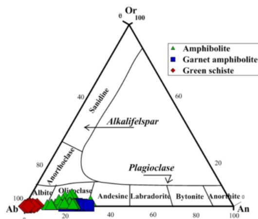
شکل ۶ نمودار مثلثی Ab-Or-An [۲۱] و برای تعیین طیف ترکیبی پلاژیوکلازهای مورد بررسی وابسته به متابازیت‌های مجموعه آذرین-دگرگونی دو چاه.
