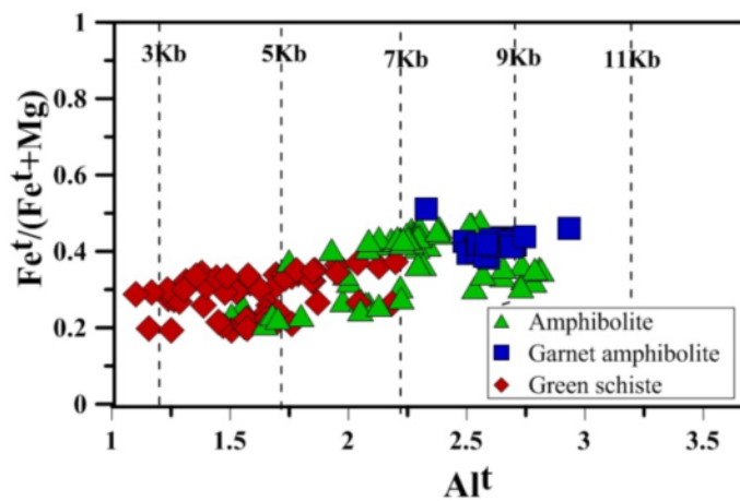
شکل ۹ نمودار Fe t /Fe t +Mg نسبت به Al t [۲۶] که فشار تشکیل متابازیت‌های مجموعه دگرگونی دو چاه را نشان می‌دهد.
