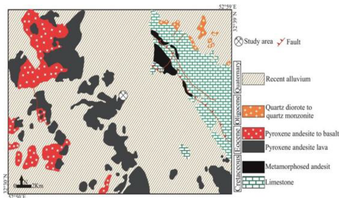
شکل ۲ نقشه زمین شناسی منطقه کالچویه (اصلاح برگرفته از مرجع [۱۷] با تغییرات)
