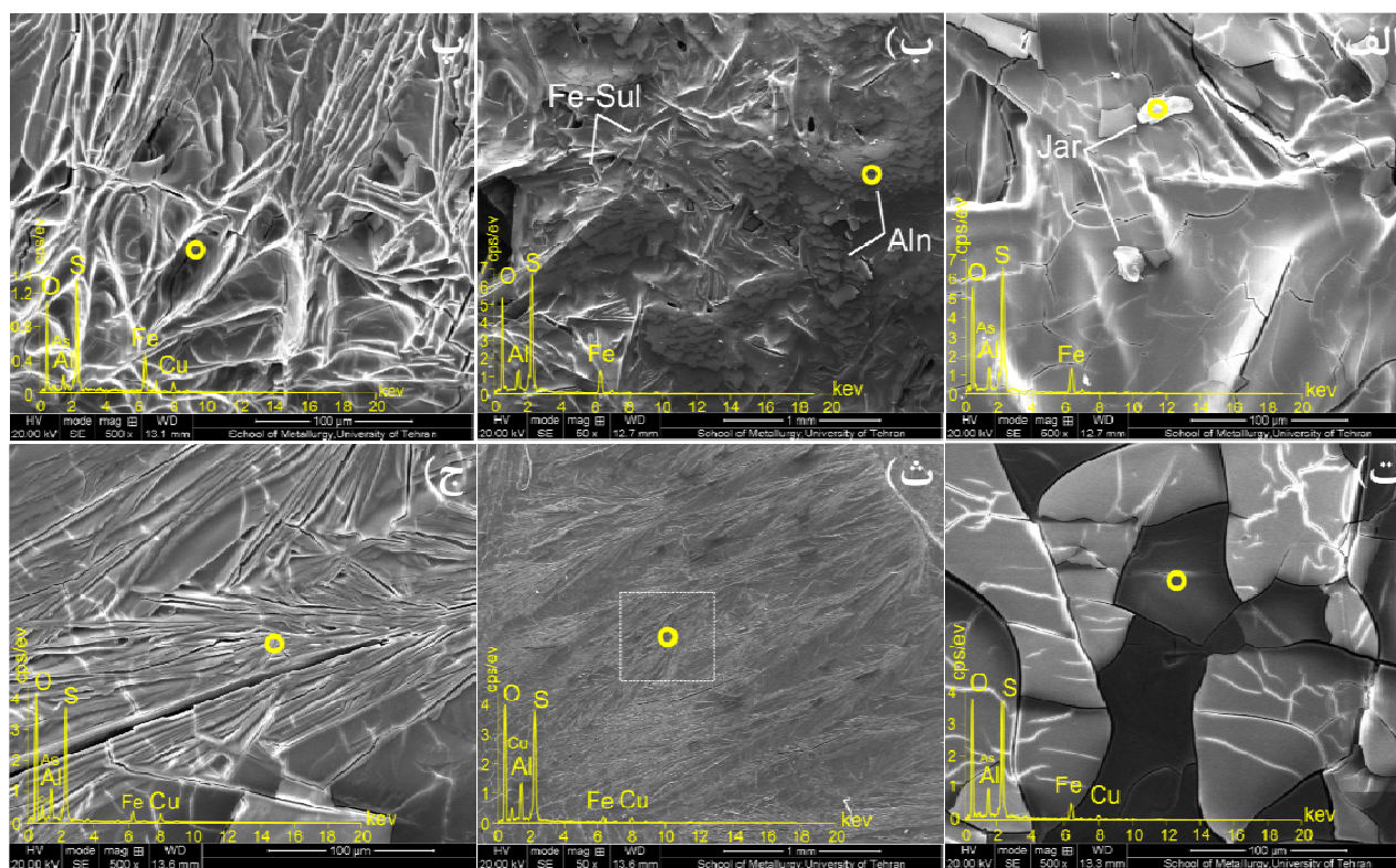
شکل ۴ تصاویر میکروسکوپ الکترونی و تجزیه شیمیایی نقطه‌ای، الف) ژاروسیت (نمونه HC1S)، ب) آلونزن (Aln) و سولفات آهن (Fe-Sul)، پ) کوکئیمبیت، ت) فری کوپاپیت، ث) سولفات‌های آلومینیم و مس. گستره مشخص شده در تصویر ج آورده شده است، ج) آنتلریت.
