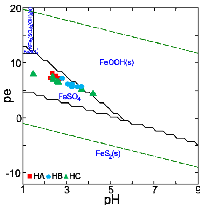
شکل ۶ نمودار \text{pe-pH} شیرابه‌های Fe-S-K-O-H برای میانگین لگاریتم فعالیت \text{Fe}^{2+} ، \text{K}^+ و \text{SO}_4^{2-} به ترتیب برابر با ۲/۲۵-، ۴/۲۱- و ۱/۹۲-.
