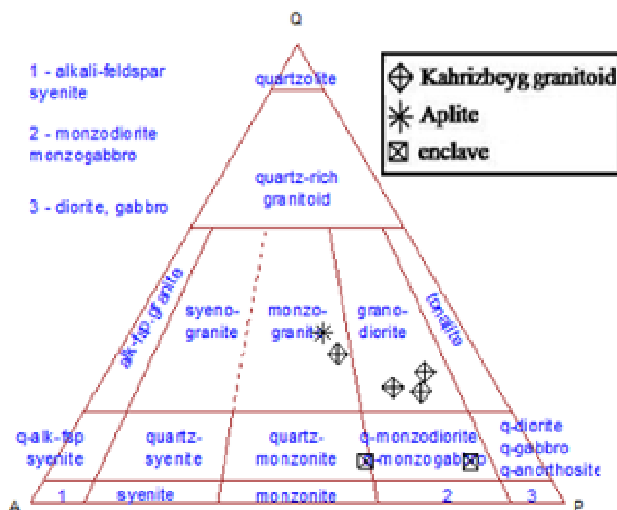
شکل ۴ نمودار رده‌بندی مودال QAP [۱۲] که نمونه‌های توده نفوذی کهریزیگ بر روی آن رسم شده‌اند.
