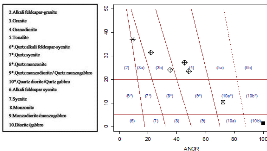
شکل ۶ نمودار Q'-ANOR [۲۸] که نمونه‌های توده نفوذی کهریزیبگ بر روی آن رسم شده‌اند. مستطیل توپر نشانگر دایک و سایر علائم مشابه شکل ۴ هستند.
