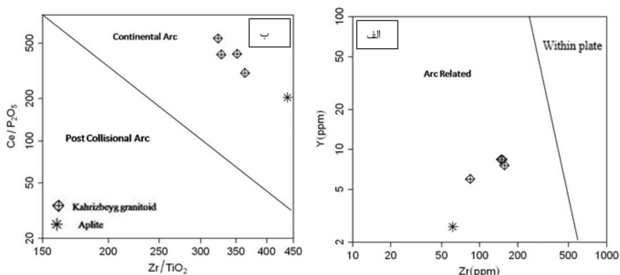
شکل ۱۷ نمودارهای تفکیک محیط زمین ساختی [۵۳] که نمونه‌های توده نفوذی کهریزیگ بر روی آنها رسم شده‌اند.
