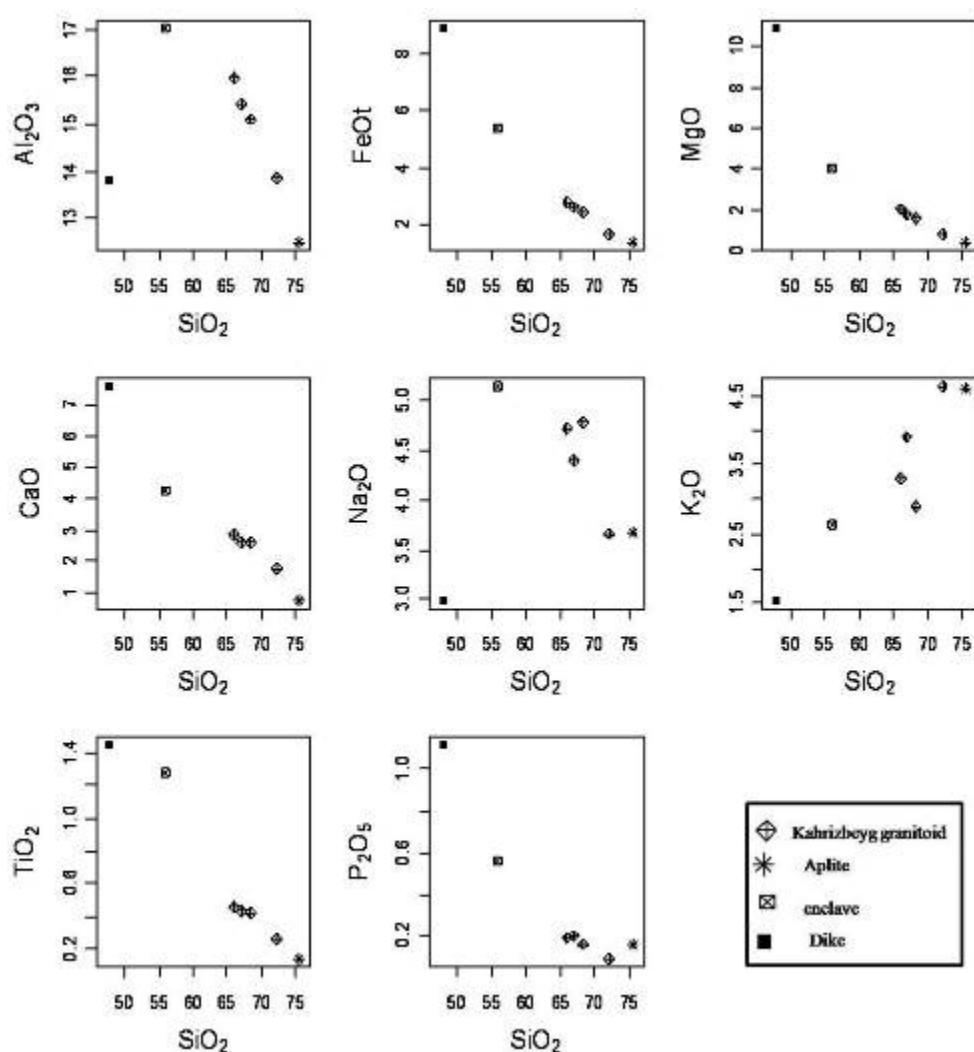
شکل ۷ نمودارهای دوتایی تغییرات اکسیدهای عناصر اصلی (wt %) و فرعی نسبت به سیلیس (wt %) [۲۹] برای نمونه‌های مورد بررسی.
