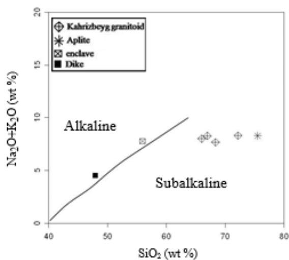
شکل ۸ نمودار مجموع قلیایی ها نسبت به سیلیس [۳۱] که نمونه‌های توده نفوذی کهریزبیک بر روی آن نشان داده شده‌اند.
